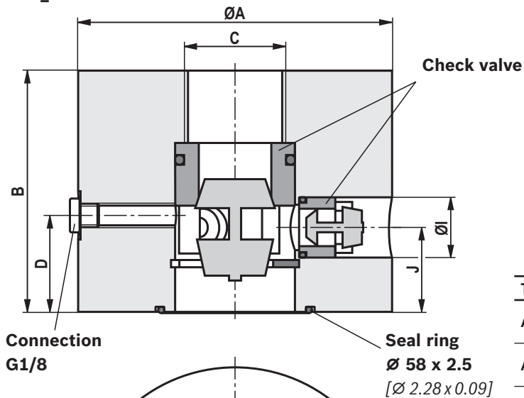
AP2_CV
